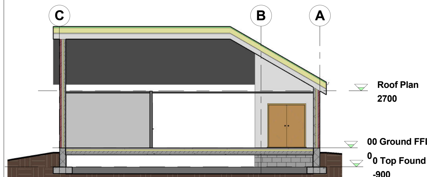
Section A-A 1 : 100
