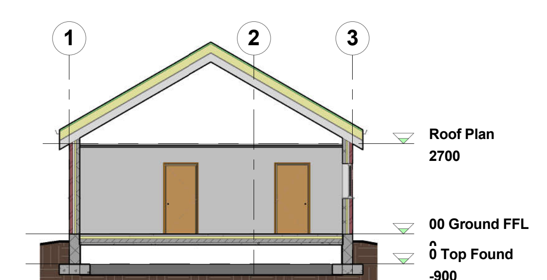
Section B-B 1 : 100
