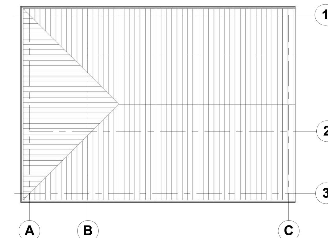
02 Roof Level 1 : 100
